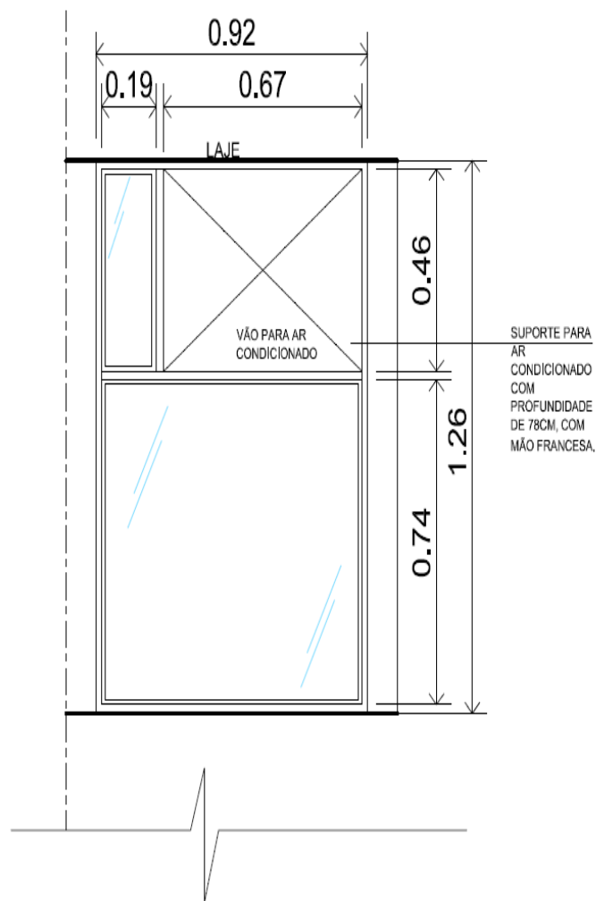
CAIXILHO 02 DO CJ. 71- VISTA FRONTAL PROPOSTO
