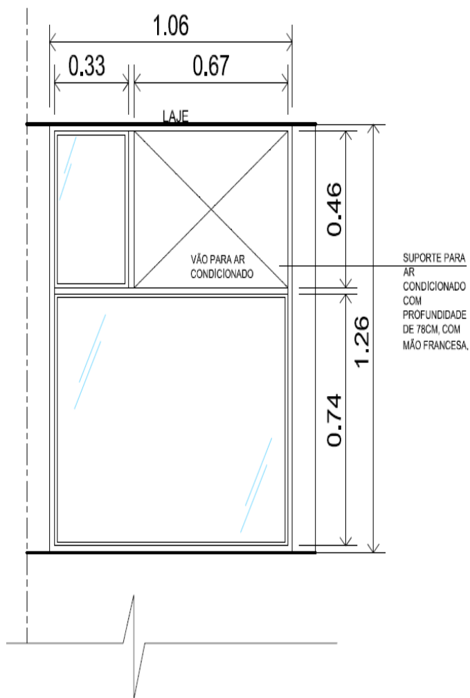
CAIXILHO 01 DO CJ. 31- VISTA FRONTAL PROPOSTO
